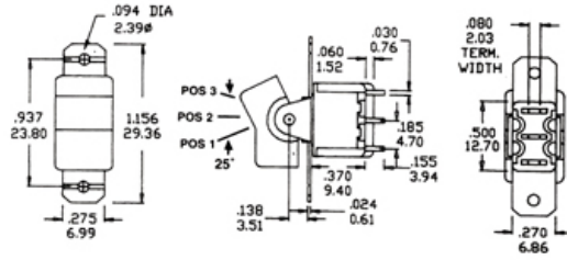
SPDT Part No.R101R1A1QN
